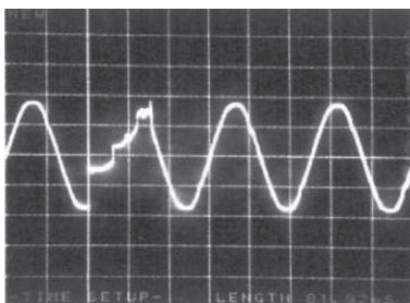
写真 1 0Ω の時 (続流発生)
