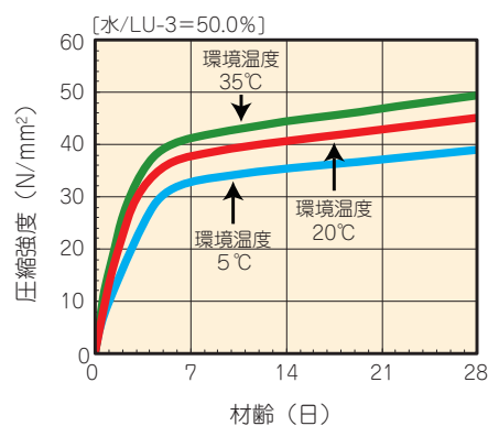
材齢と圧縮強度の関係
