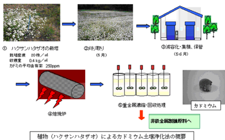
図-6 カドミウム・亜鉛の吸収及び回収方法の概要
