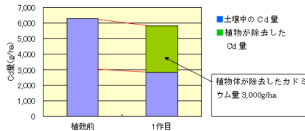
図-1 ハクサンハタザオを屋外で1作栽培した前後の土壌Cd濃度の変化
