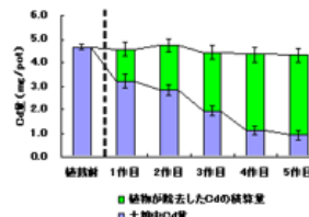
図-5 Cd収支(ポット)
