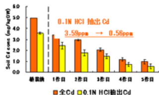
図-4 土壌中Cd濃度の変化(ポット)
