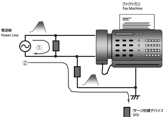
図4 サージ防護デバイスの対策方法 Fig.4 Example of Surge Protection
