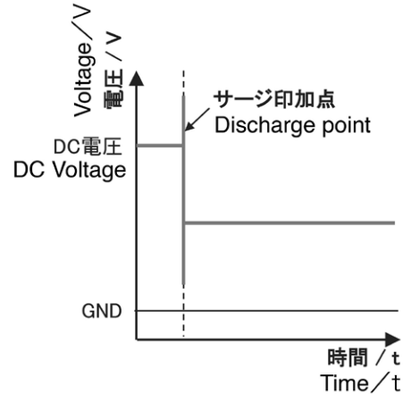
図11 ホールドオーバーの発生 Fig.11 Holdover occurring
