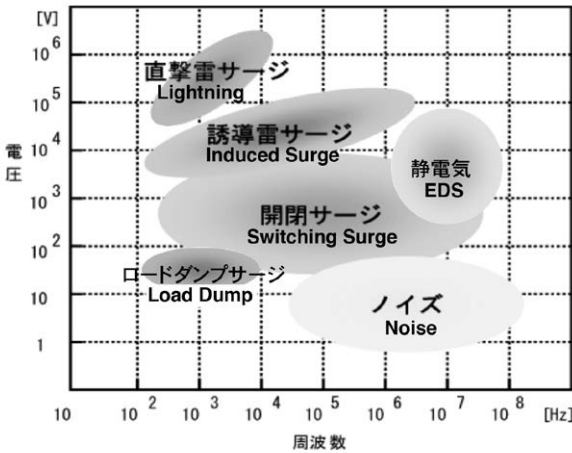
図1 サージの種類 Fig.1 Surge Types
