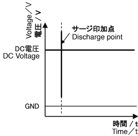
図10 ホールドオーバーの発生無し Fig.10 No Holdover occurring
