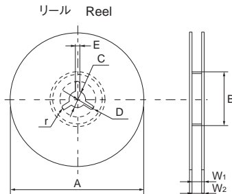
プラスチックリール (標準型) Reel 単位 unit (mm)
