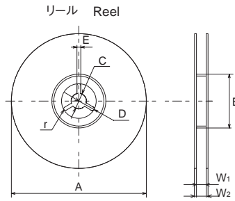
プラスチックリール (標準型) Reel 単位 unit (mm)
